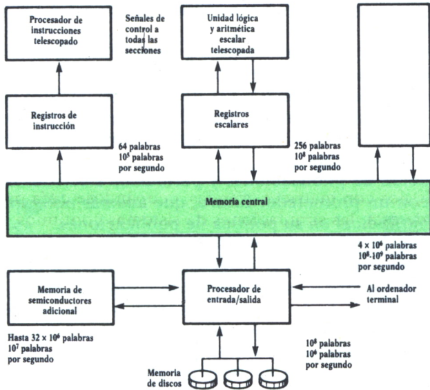
Fig. 6. Ejemplo de ordenador paralelo multiprocesador.
