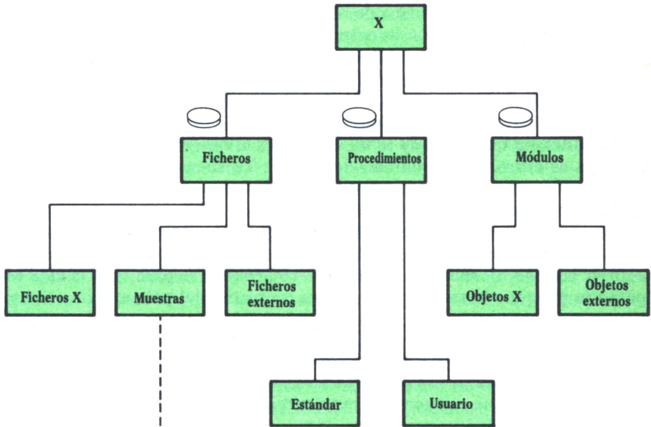
Fig. 5. Sistema real de ficheros.
