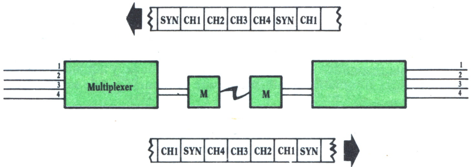
Fig. 8. Multiplexación en el tiempo.
